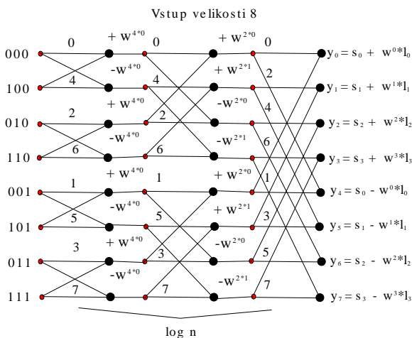
Příklad průběhu algoritmu pro vstup velikosti 8
